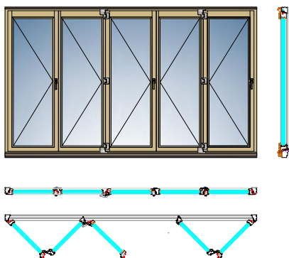
FS-портал-гармошка. Схема 532
