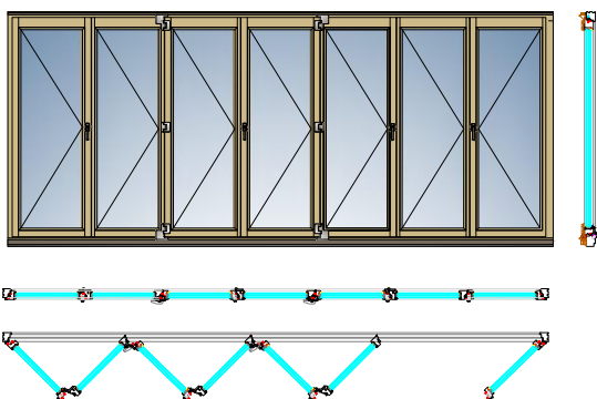
FS-портал-гармошка. Схема 761 (6+1)
