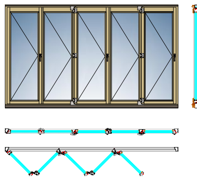
FS-портал-гармошка. Схема 550
