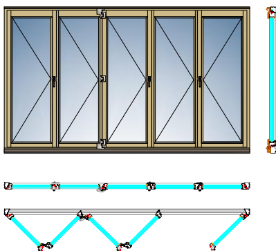
FS-портал-гармошка. Схема 541
