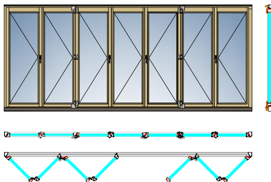
FS-портал-гармошка. Схема 743*
