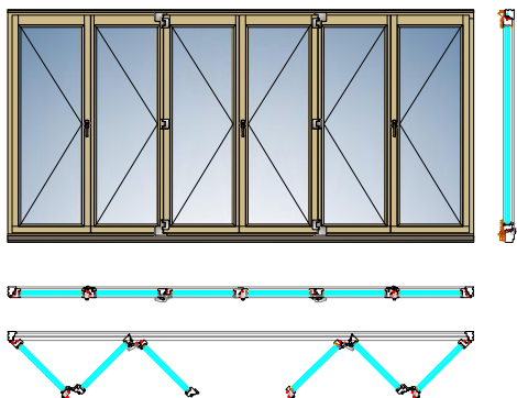
FS-портал-гармошка. Схема 633 (3+3)
