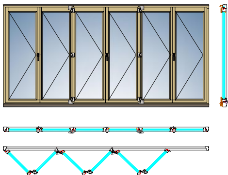
FS-портал-гармошка. Схема 660*
