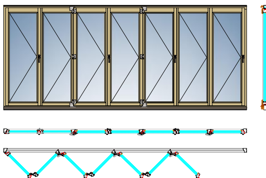
FS-портал-гармошка. Схема 770*
