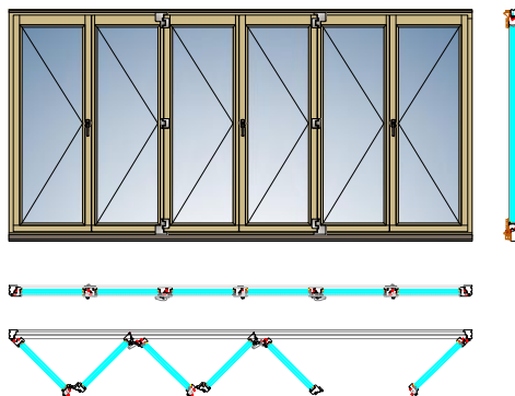
FS-портал-гармошка. Схема 651 (5+1)
